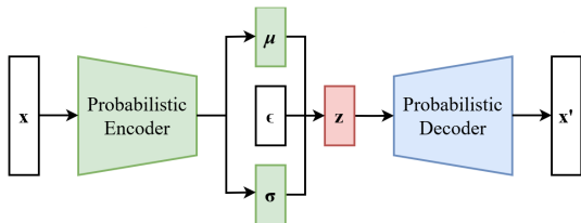
Figure 4 – Schéma d'« Auto-encodeur variationnel », 2024
